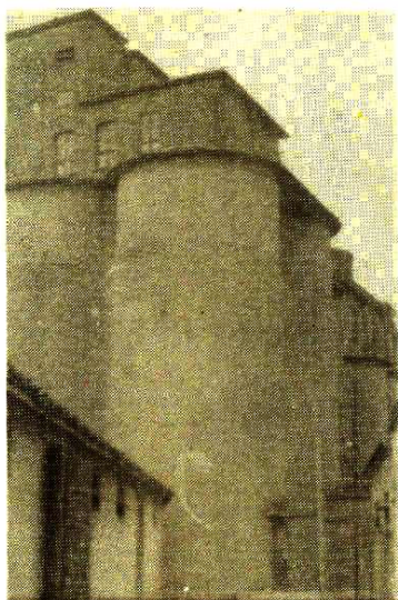
砖筒仓(面粉车间)
