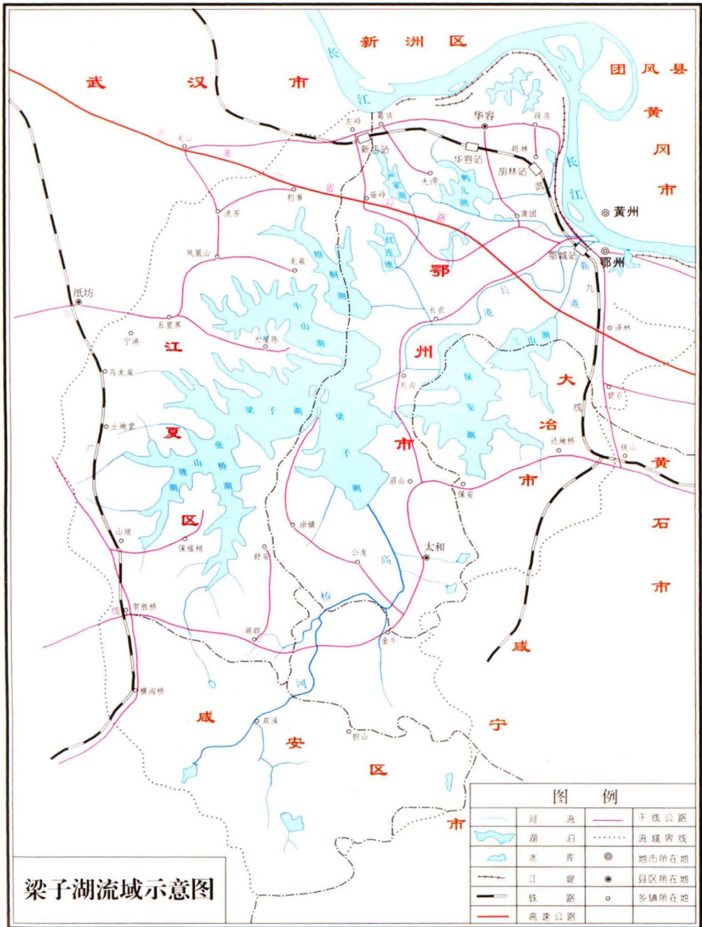
梁子湖流域示意图
