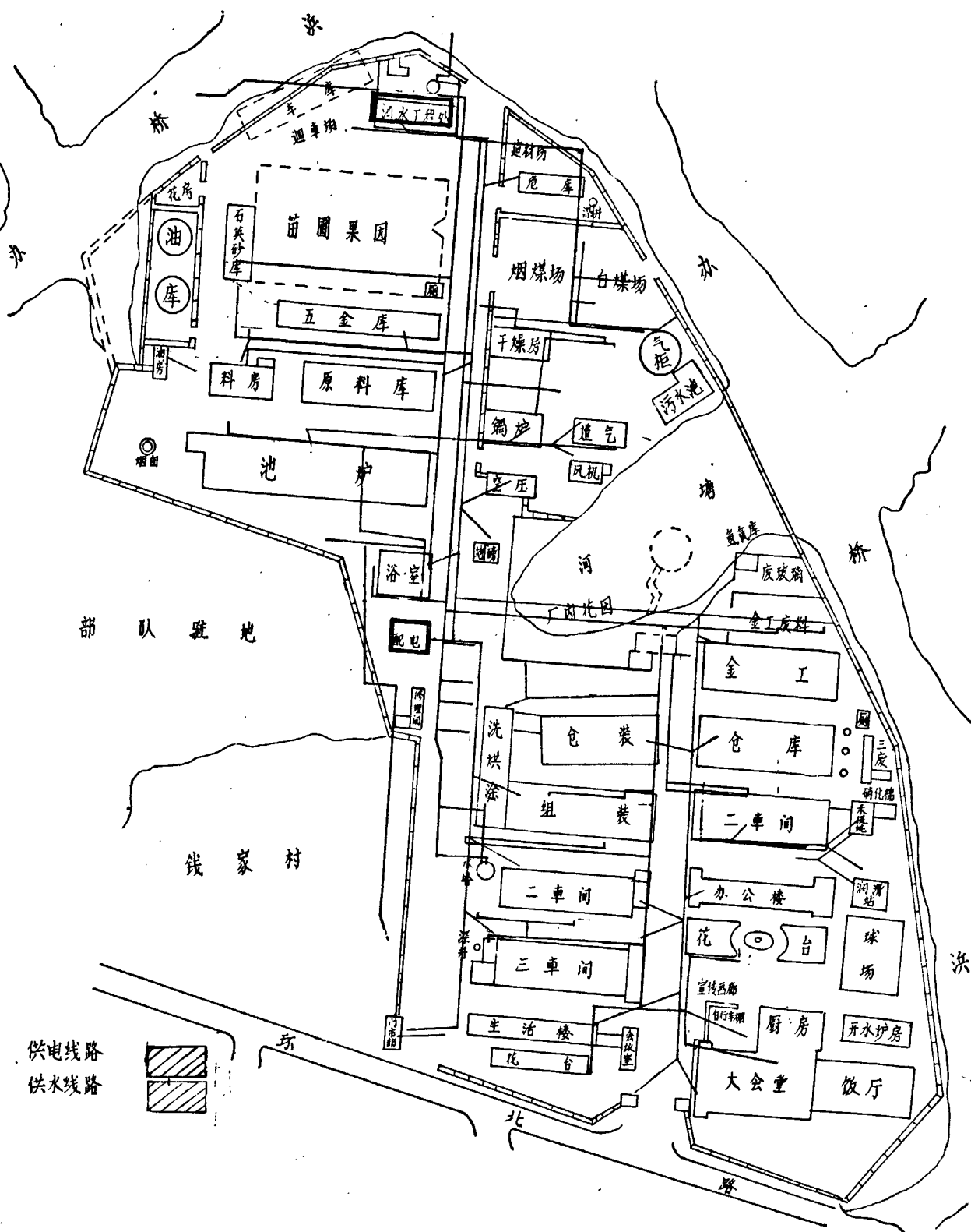
供电、供水线路图
