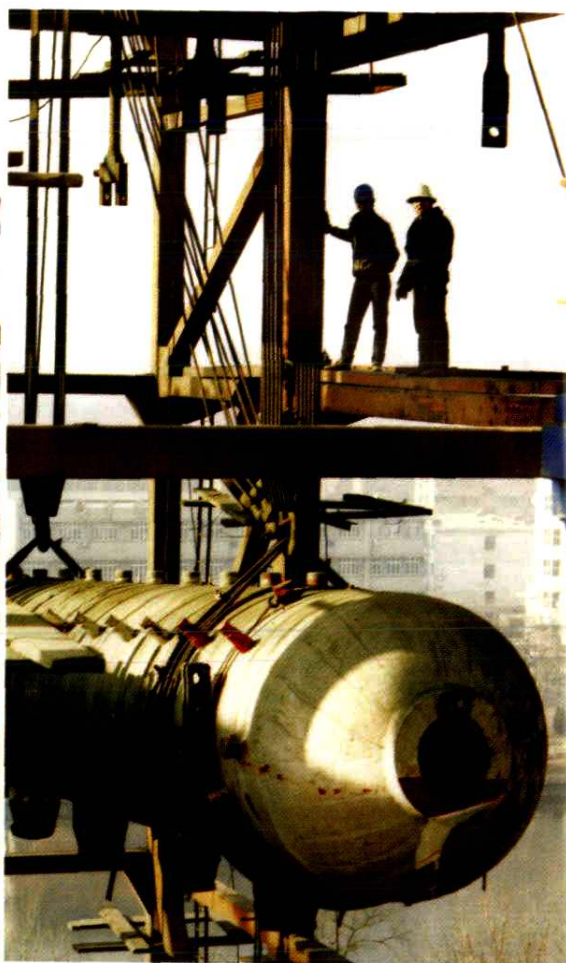
天津第一热电厂扩建工地锅炉汽包吊装
