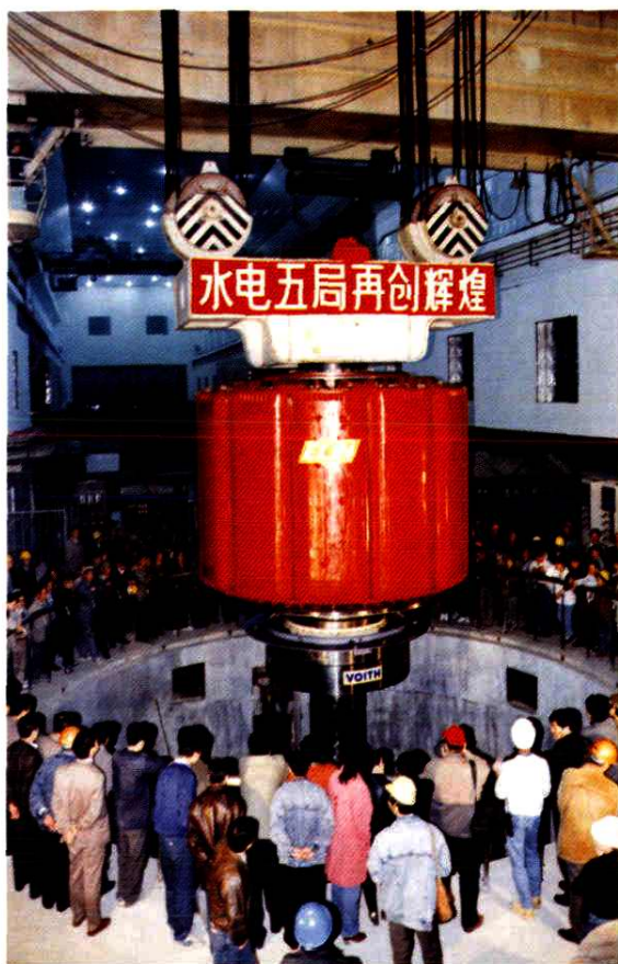
十三陵抽水蓄能电站 200 兆瓦水轮机转子吊装
