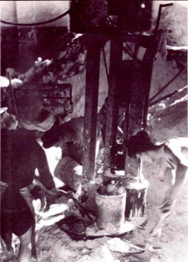
①冲盐机冲盐 ②自制脚踏卷扬机 ③人工翻矿 ④高压水冲碇 ⑤人 工冲盐
