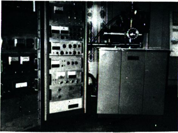
△俄歇电子谱仪
