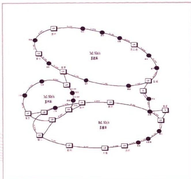
⑦ 1998年省内长途传输SDH环网络结构图
