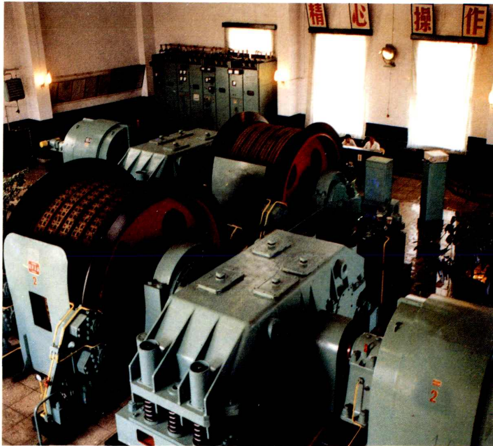
主井絞車房
