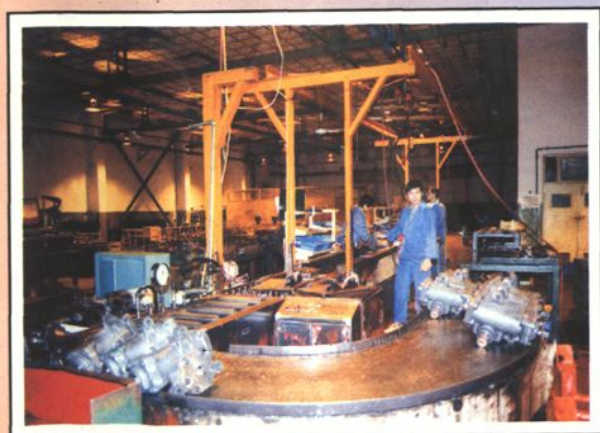
动力转向器总成装配线
