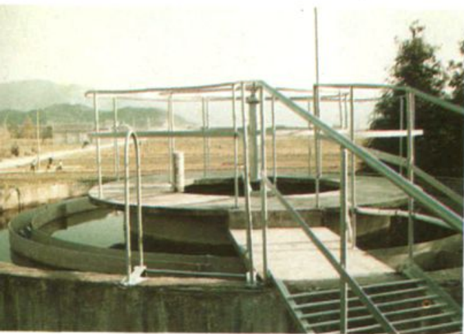
龙场水厂改进型水力循环澄清池
