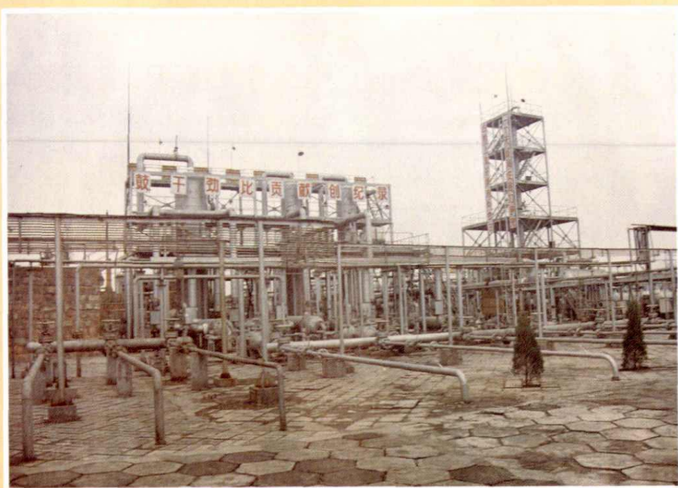
▲ 低温分离集气站
