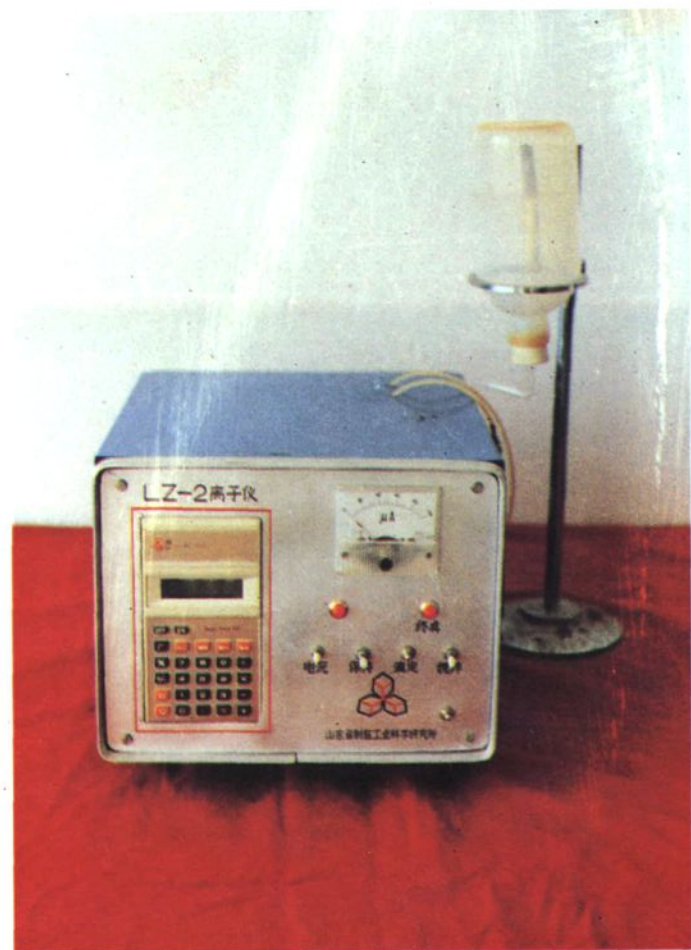
我所研制的LZ-2型离子仪
