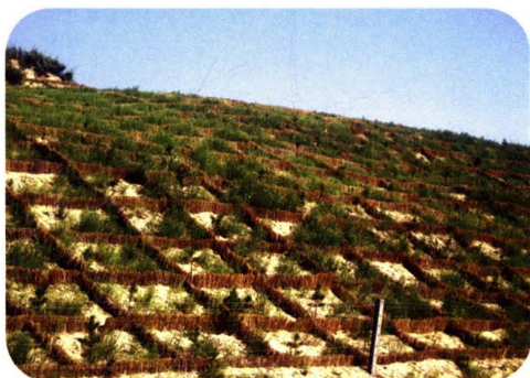
机械沙障
