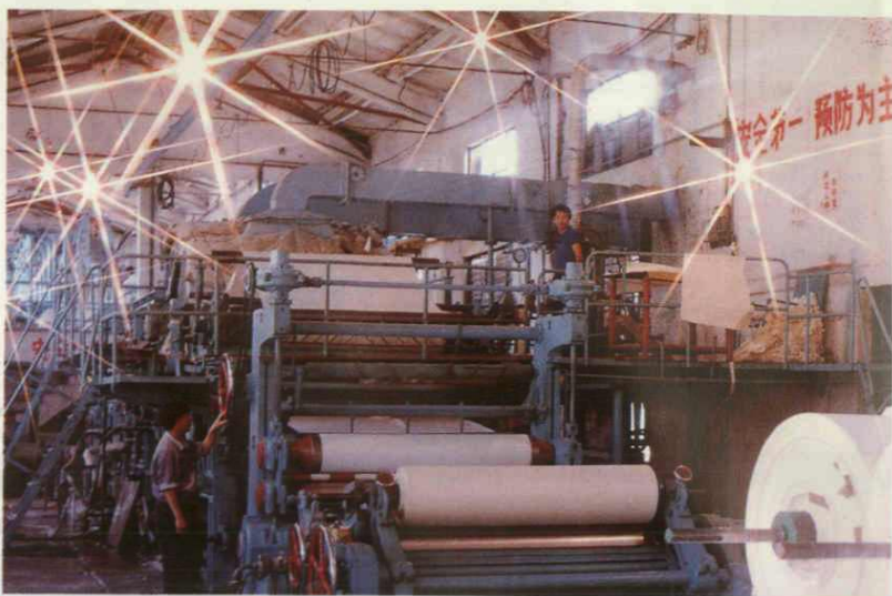
机制纸生产线一角
