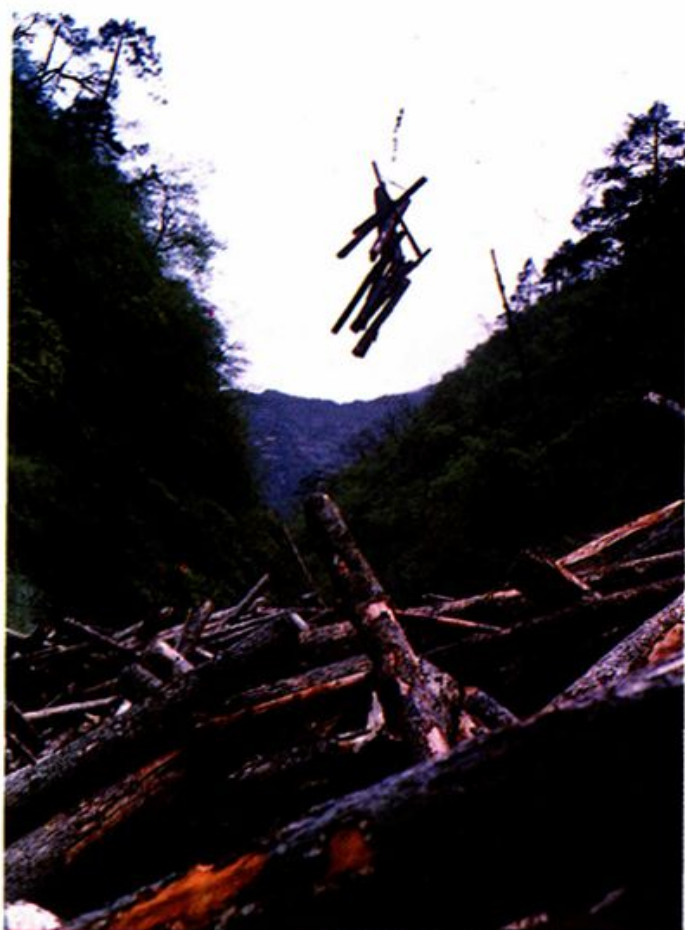
◀ 架空索道集材
