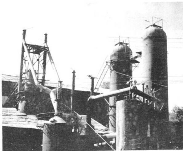
宣威县田坝镇炼铁厂的考贝式热风炉
