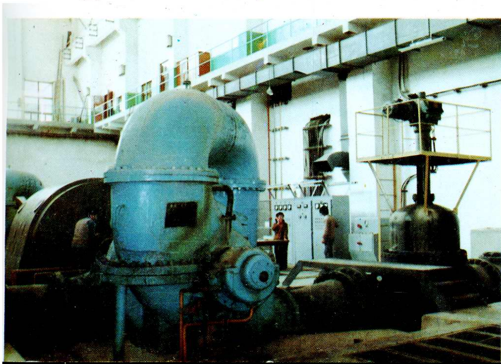
东雷二级站机组
