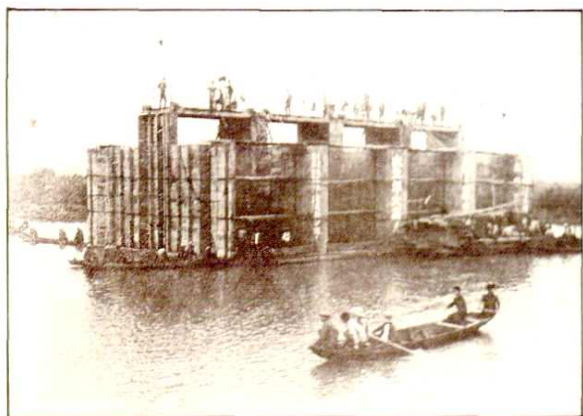
东河口水闸施工时，第一座浮运闸拖运场面。
