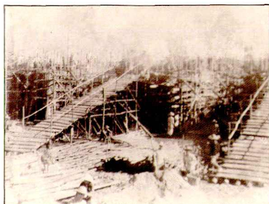
当年西河口水闸施工现场一角。
