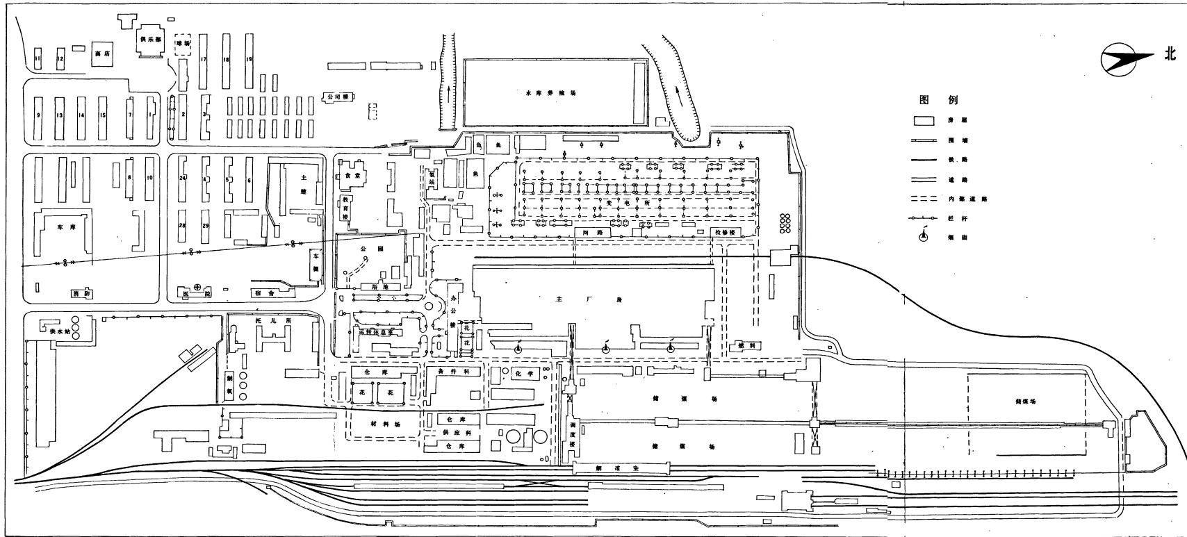
辽宁发电厂厂区平面图 1985年
