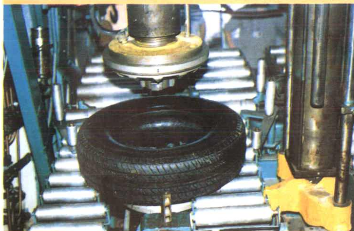
◀四川橡胶厂子午轮胎 X 光机检测
