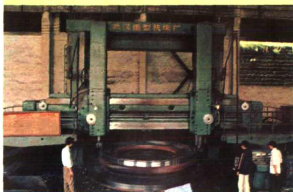
▲四川省建材机械厂采用 C5250-1, 5M 立式车床加工水泥生产设备
