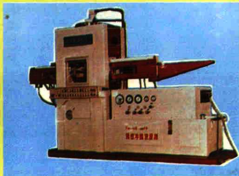
▲内江锻压机床厂产的 Y26 - 100 型 1000 千牛精密冲裁液压机
