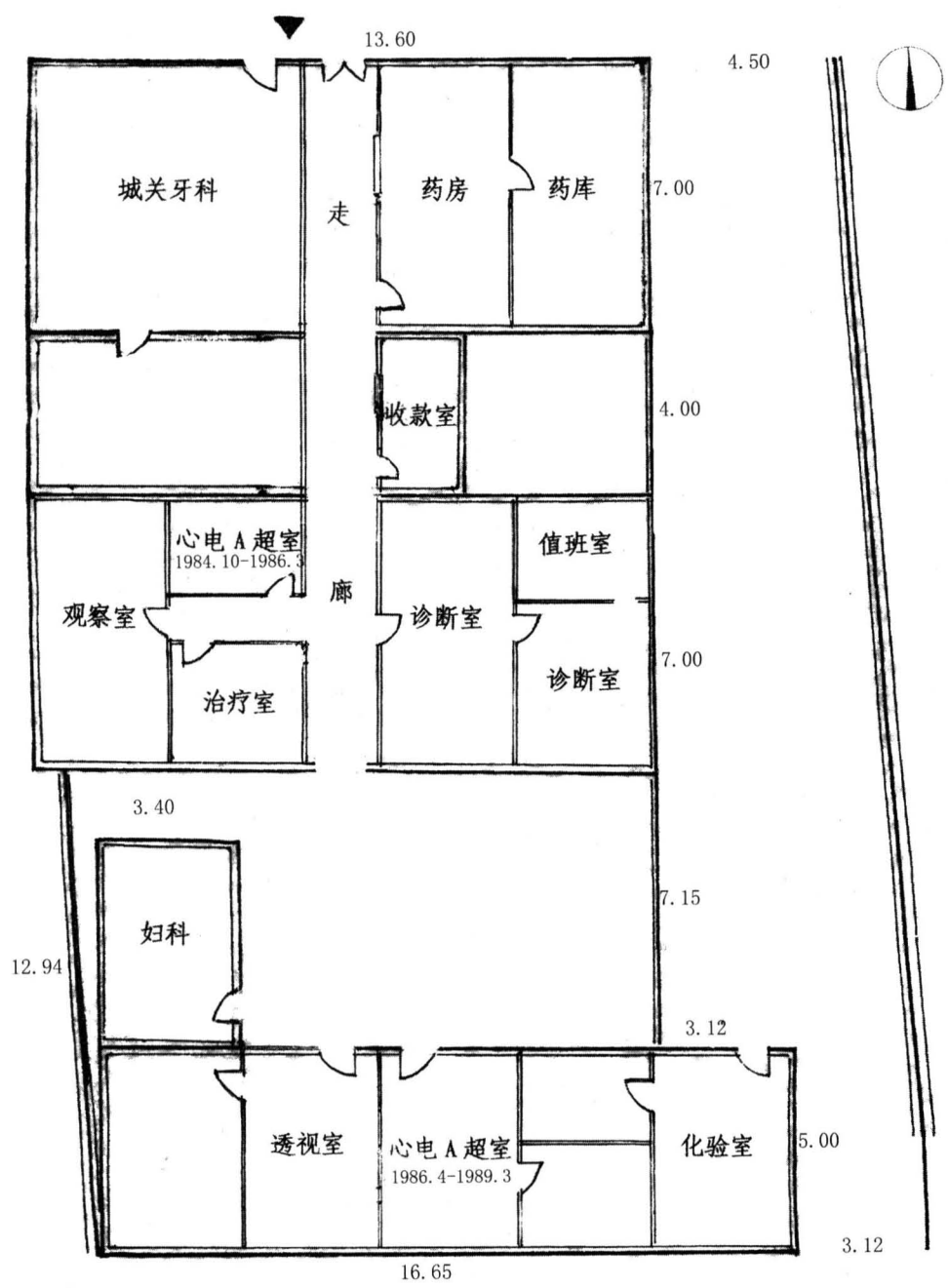
平度县中医院独立之初平面示意图
