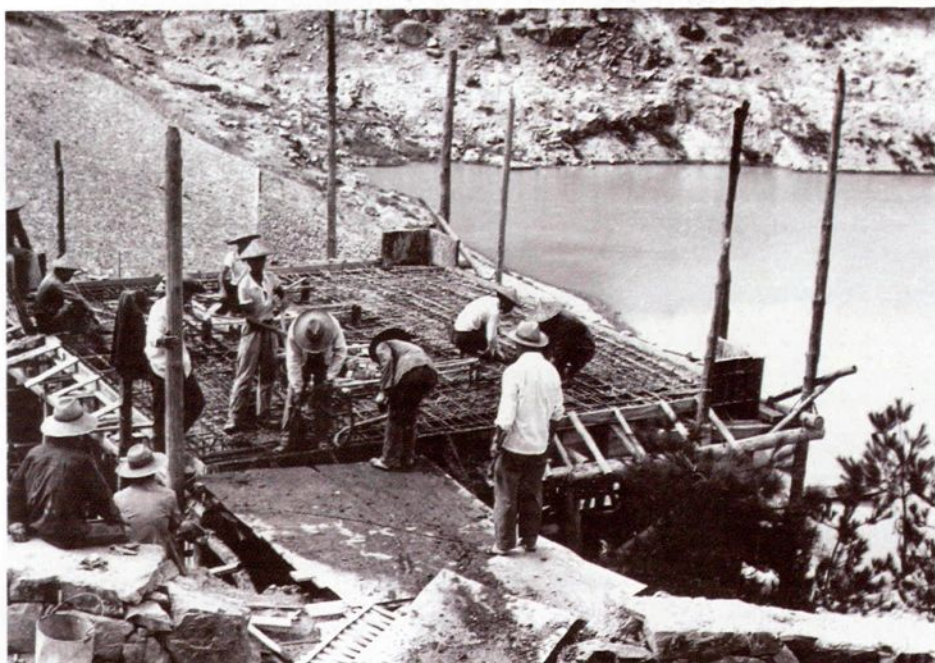
钟前水库泄洪闸启闭机台在施工中(1987年9月4日)
