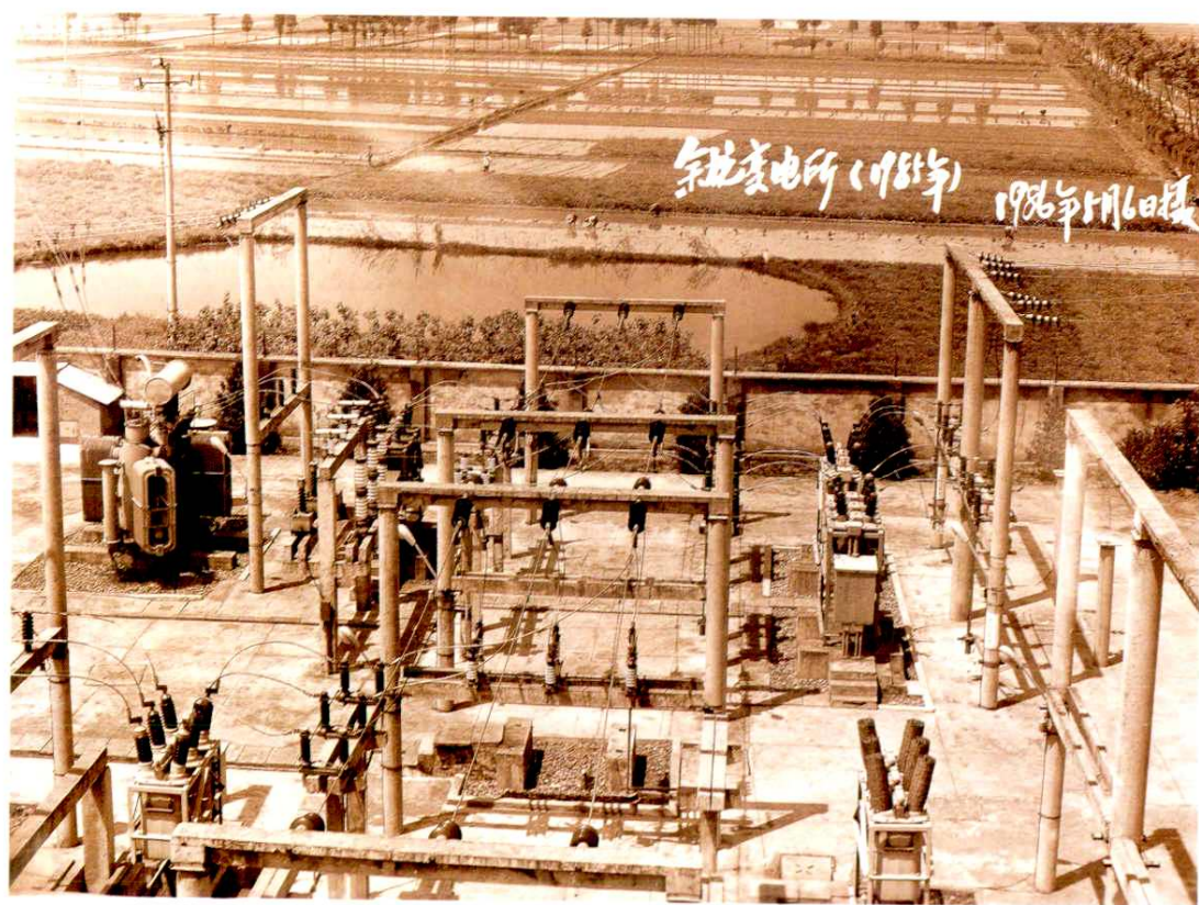
建于1985年的35千伏余杭变电所
