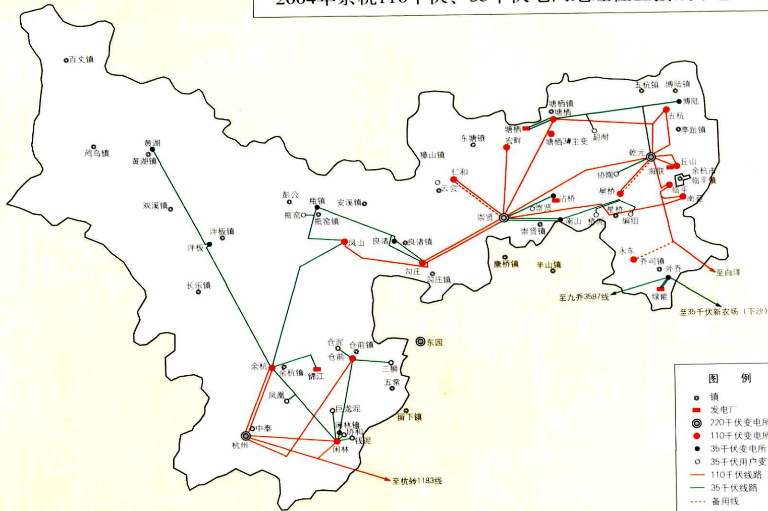
2004年余杭110千伏、35千伏电网地理位置接线示意图
