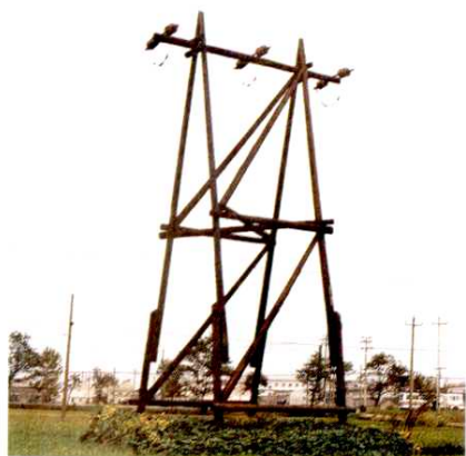
全省第一条35千伏输电线路(杭海线)
