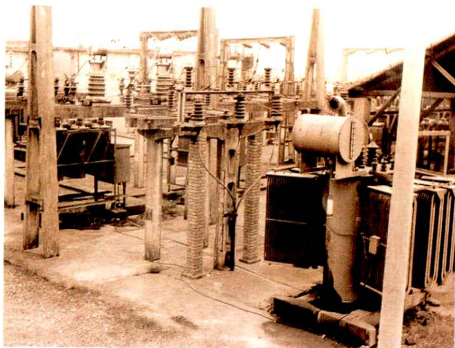
建于1957年的余杭首座35千伏临平变电所
