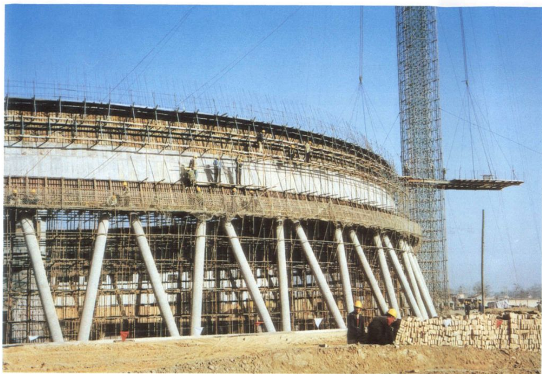
18、1992年3~10月，蒲电1号冷水塔环梁浇灌砼紧张施工
