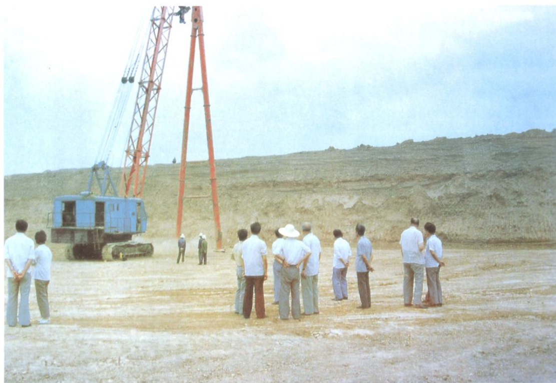
17、1989年6月，蒲城电厂建设公司经理陪同上级领导在主厂房基坑内查看施工机械
