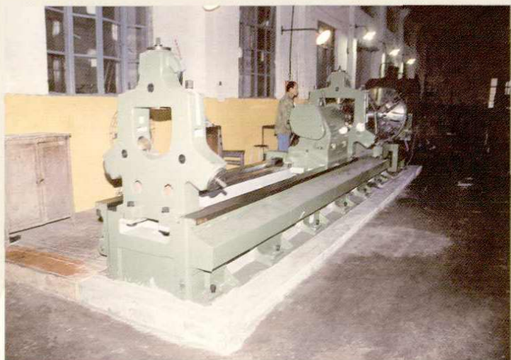
上海华泰机械厂的 C61100 车床。
