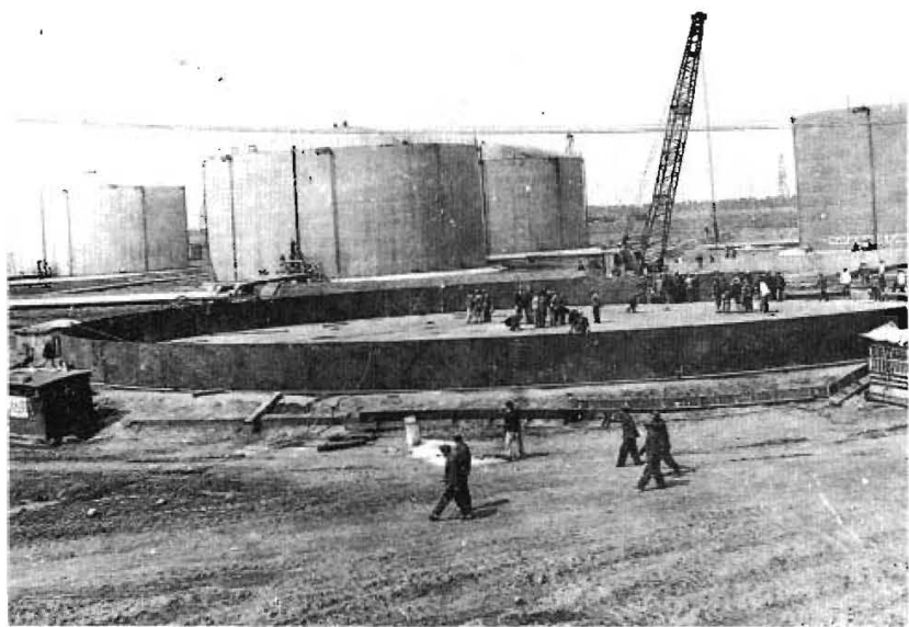
建设中的任丘油田北大站
