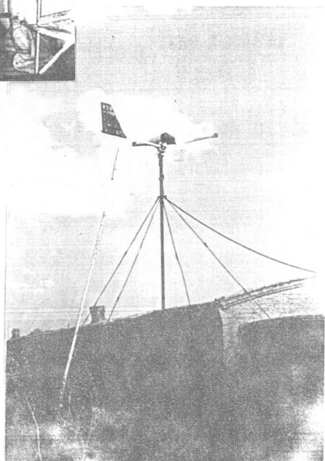
家庭小牧场风力发电机
