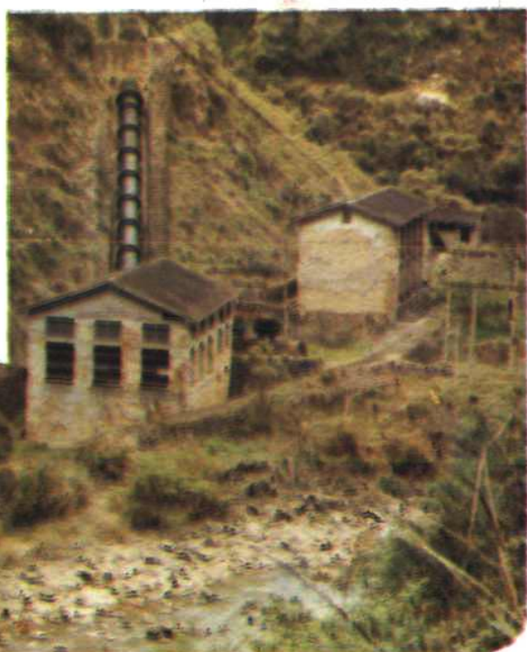
▲掬秀潭水电站外观
