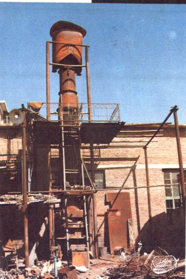
一九八一年六月锦州市总工会群众技术协作委员会帮助锦州液压件厂改成的冲天炉
