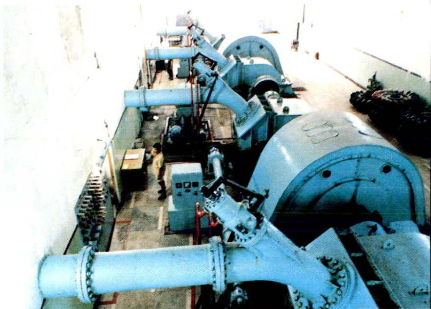
百丈 漂电厂一级站水轮发电机组
