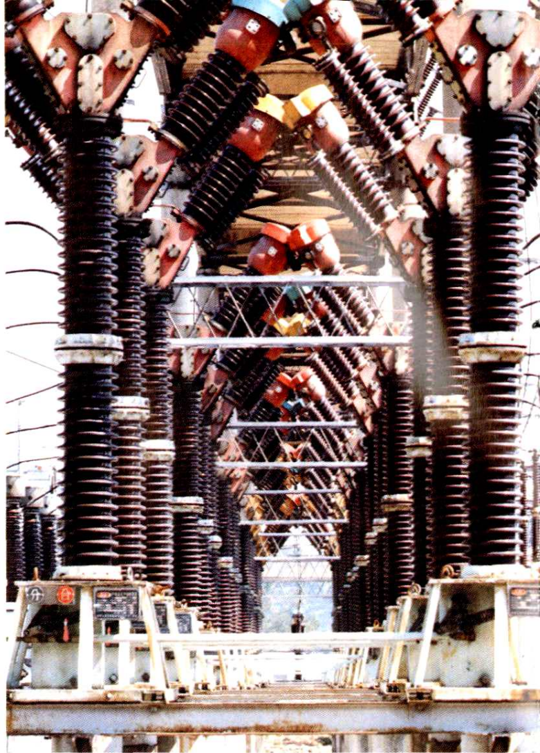
慈湖变电所开关设备
