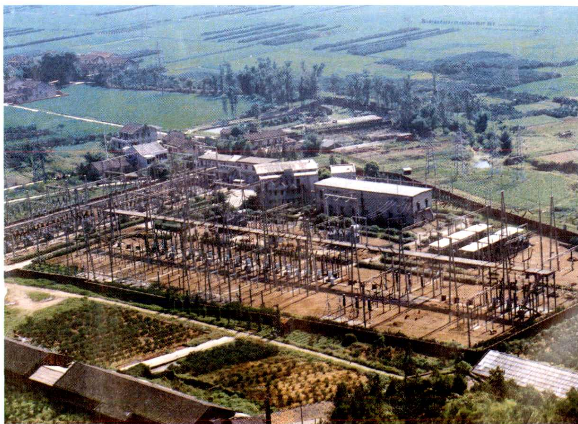
220 千伏慈湖变电所俯瞰
