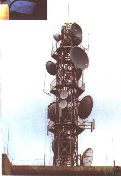
楚雄州广播电视局 于 20 世纪 90 年代中期 建成的楚雄州广播电视 微波网紫溪山中枢站微 波天线塔
