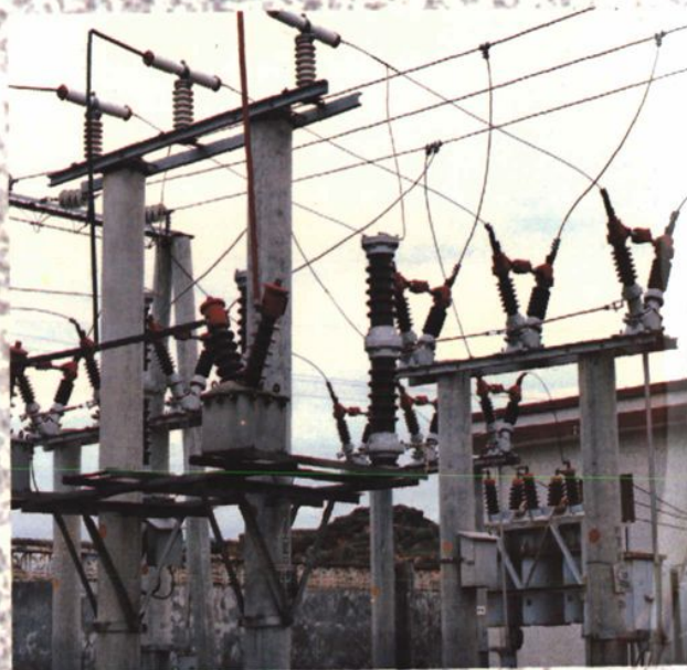
长福变电站
