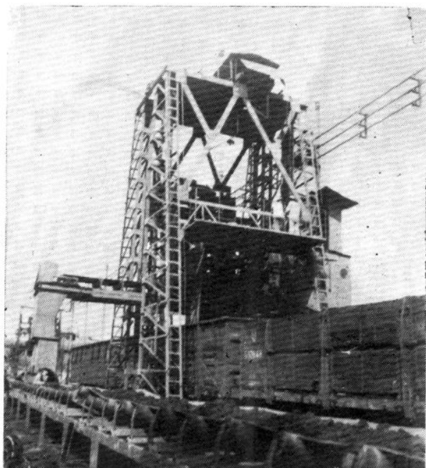
▶ 自制卸煤机
