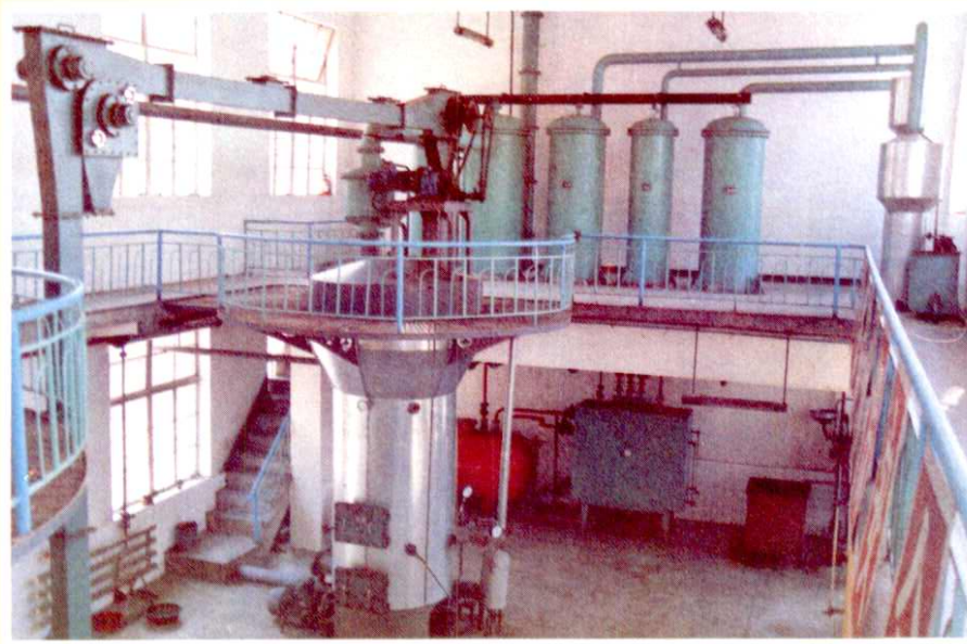
(图 6-17)浸出油车间层碟式汽提塔
