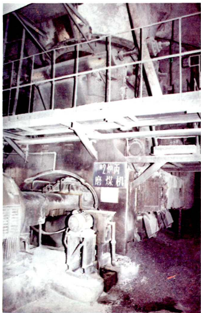
二十一、平盘中速磨煤机
