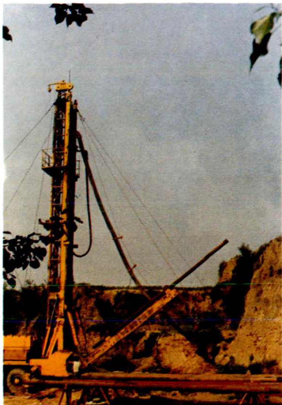
水文地质局从法国引进的 RH-28 型全液压车装水井钻 机，在太行山区施工
