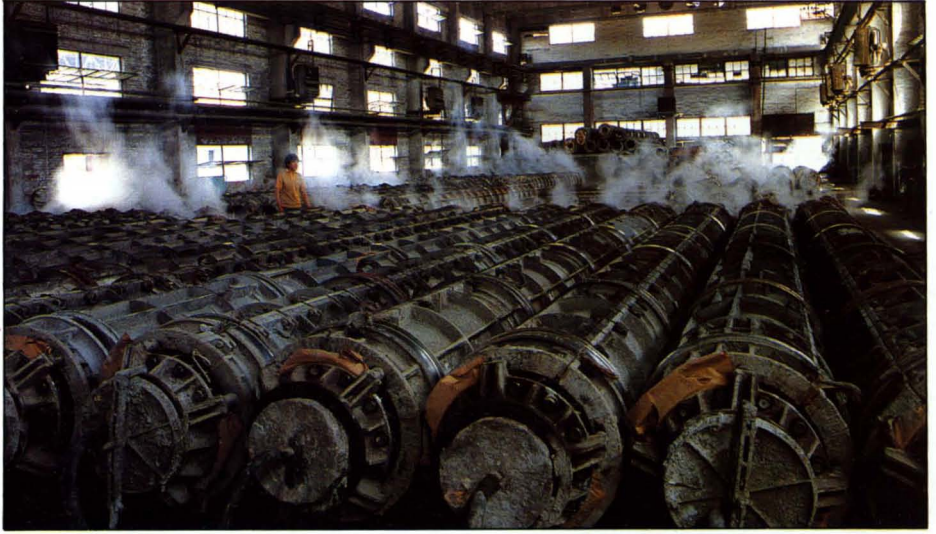
生产车间正在进行 预应力混凝土管桩 的蒸汽养护。
