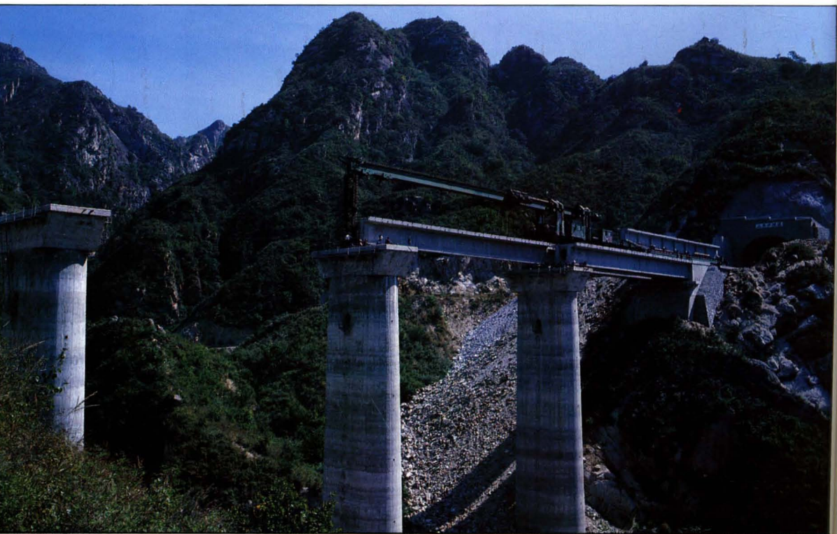
1987年，正在架设中的大秦线铁路桥梁。
