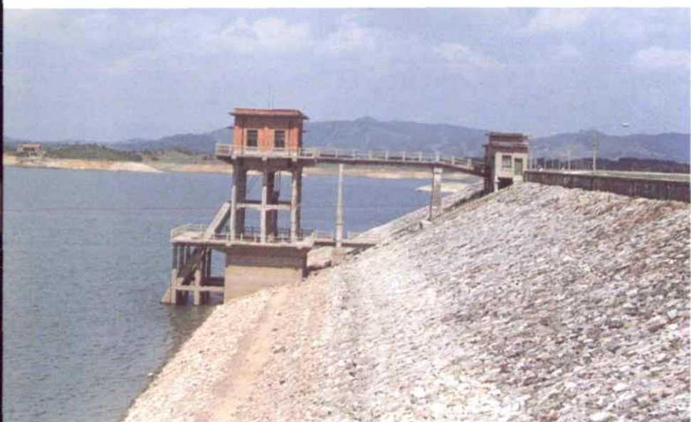
输水洞进口
