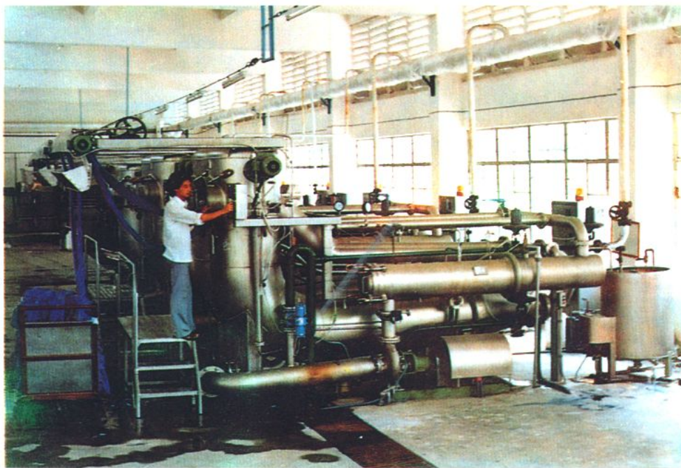
开平县针织厂染整车间高温高压染色机
