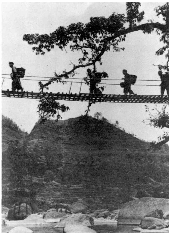
左图：歇马公社石洞槽铁索桥。
