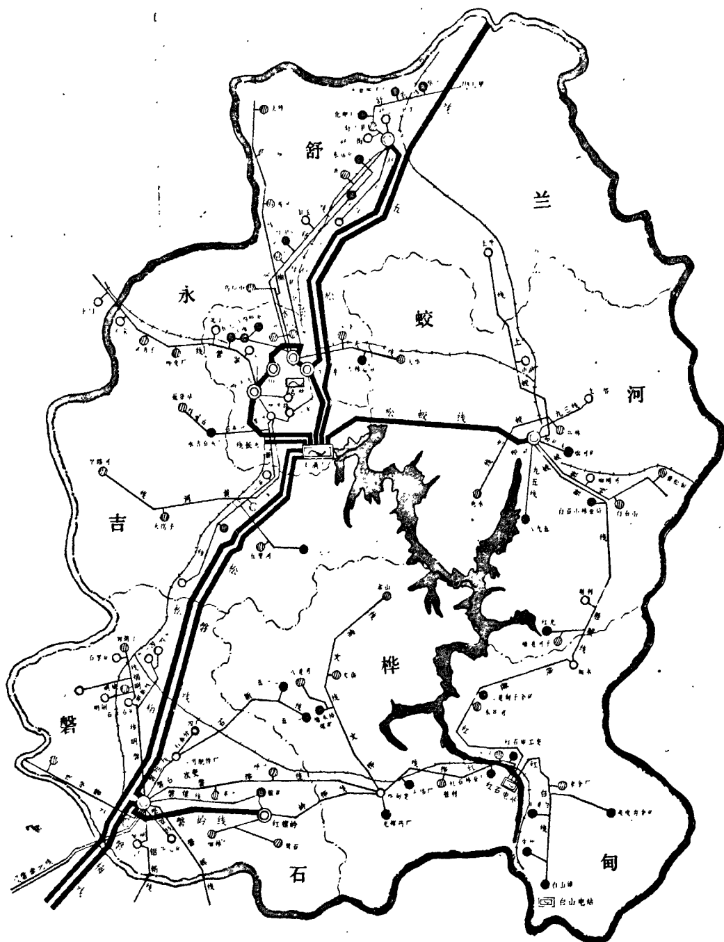
吉林地区电力系统地理位置图
