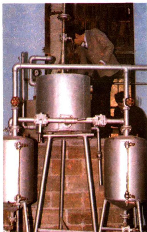
岑巩香料厂山苍子油生产流程塔
