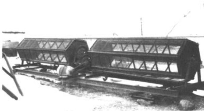
奇克粮库自制的大豆电动清选机
