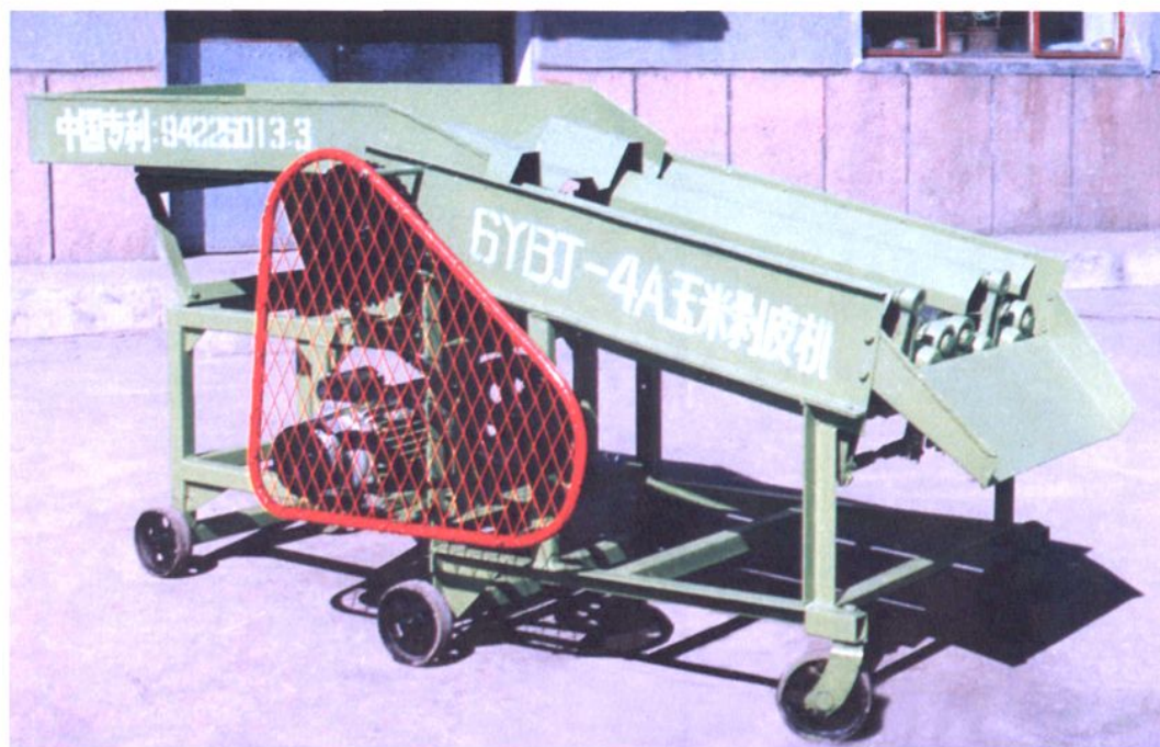
6YBJ-4A 玉米剥皮机
