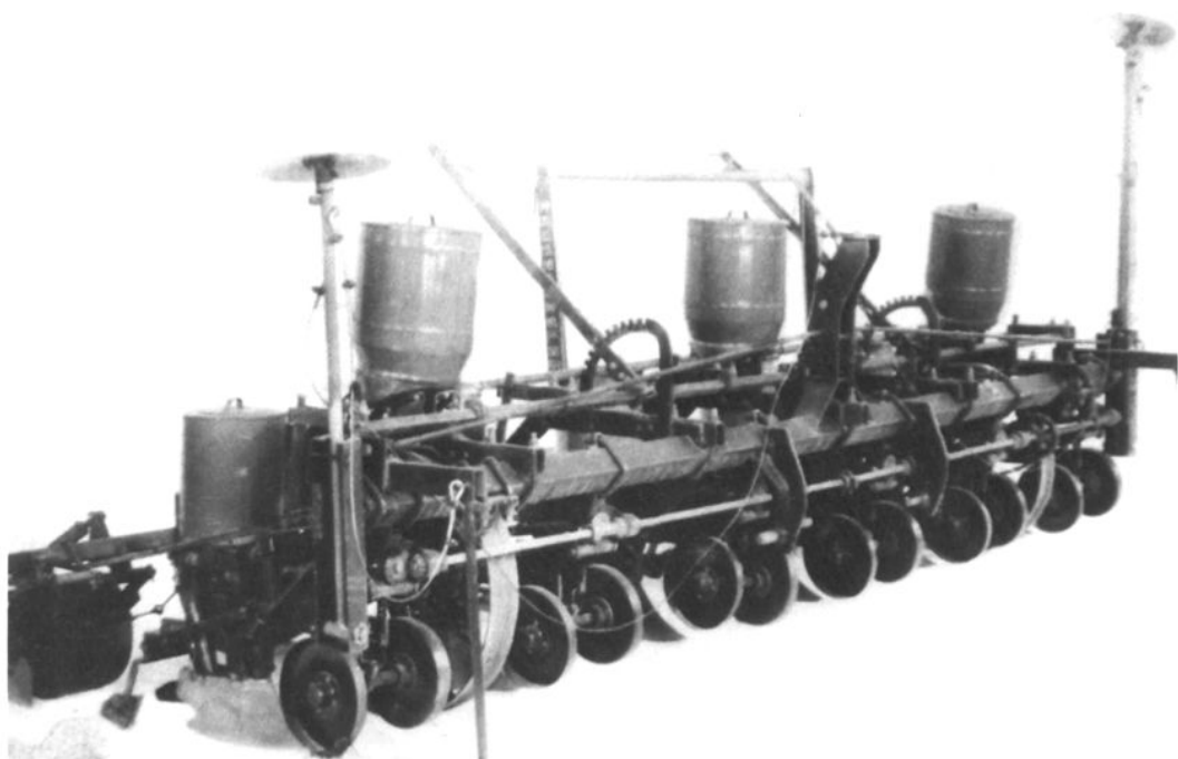
BZ-6 综合号播种机 (1983 年获国家发明三等奖)
