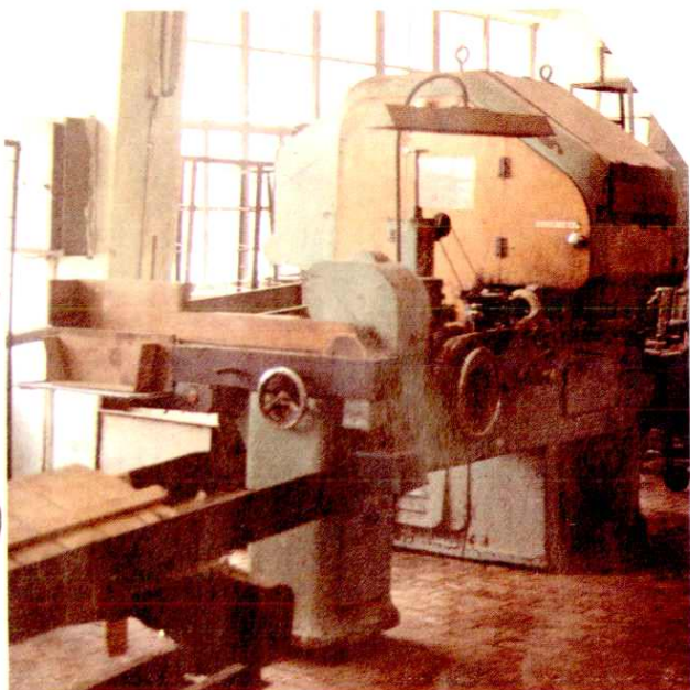
▲ 1983年前使用的 YJ — 11 卷烟机 (赣南机械厂造)
