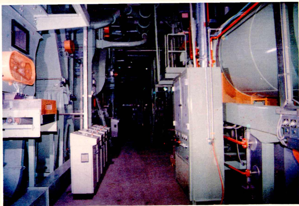
▲ 以八千多万元巨资引进的意大利科马斯 (COMAS) 现代化制丝设备
