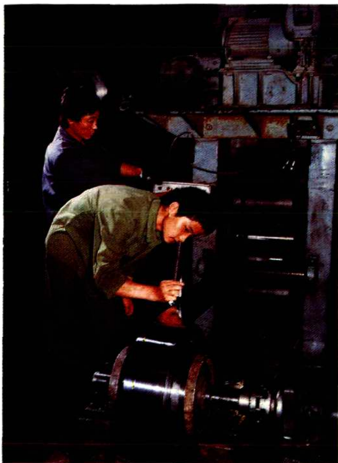
沧州市轧钢厂的四 辊轧钢生产线正在轧制 钢带
