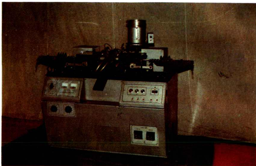
市通用机械厂生产的高速电阻引线对焊机
