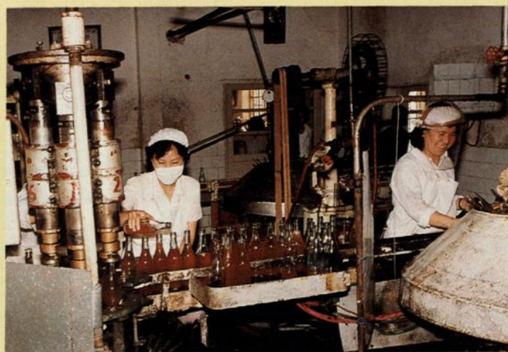
用好政策，促進生產發展。圖為縣食品廠汽水生產車間。
