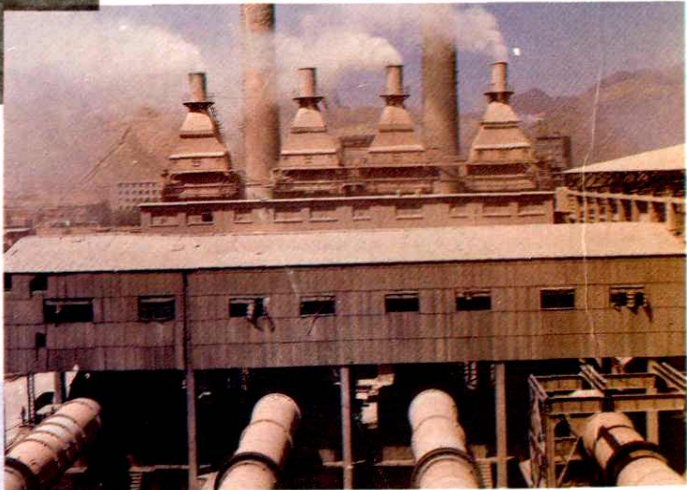
50 年代从民主德国全套引进的永登水泥厂 4 条湿法回转窑水泥生产线
