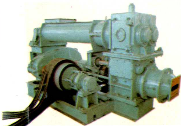
兰州建材机械厂自行设计制造的挤砖机、挤瓦机
