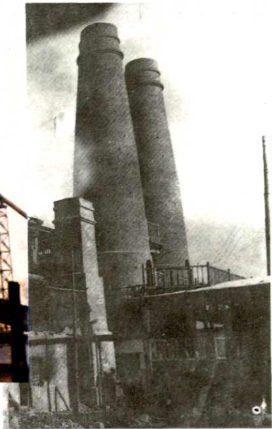
甘肃水泥公司超福氏大窑及胜利式小窑（1942 年）和在其原址建成的窑街水泥厂年产 20 万吨的窑外分解干法回转窑生产线（1986 年 6 月）
