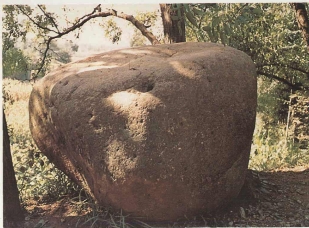
彭县塔坪漂砾
