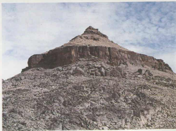
彭县太子山飞来峰——海拔4900米 何银武摄
