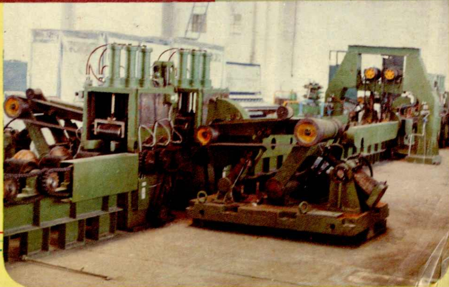
苏州冶金机械厂生产的 部优质产品中速中负荷 钢坯修磨机
