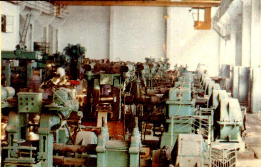
苏州铜材厂设计能力 为年产4000吨的第三 代铜皮车间
