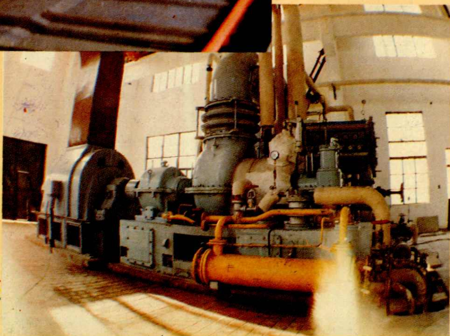
吴县钢铁厂1500kw 余热电站
