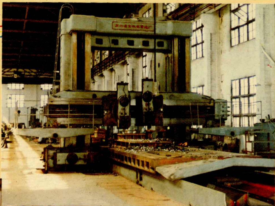
苏州冶金机械厂的 3 \times 8 \text{ m} 龙门刨
